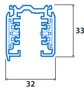
DALI 3-Circuit
